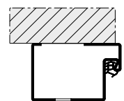
Ościeżnica blokowa montowana do ściany (profil 006) (badana po stronie bez zawiasów)
