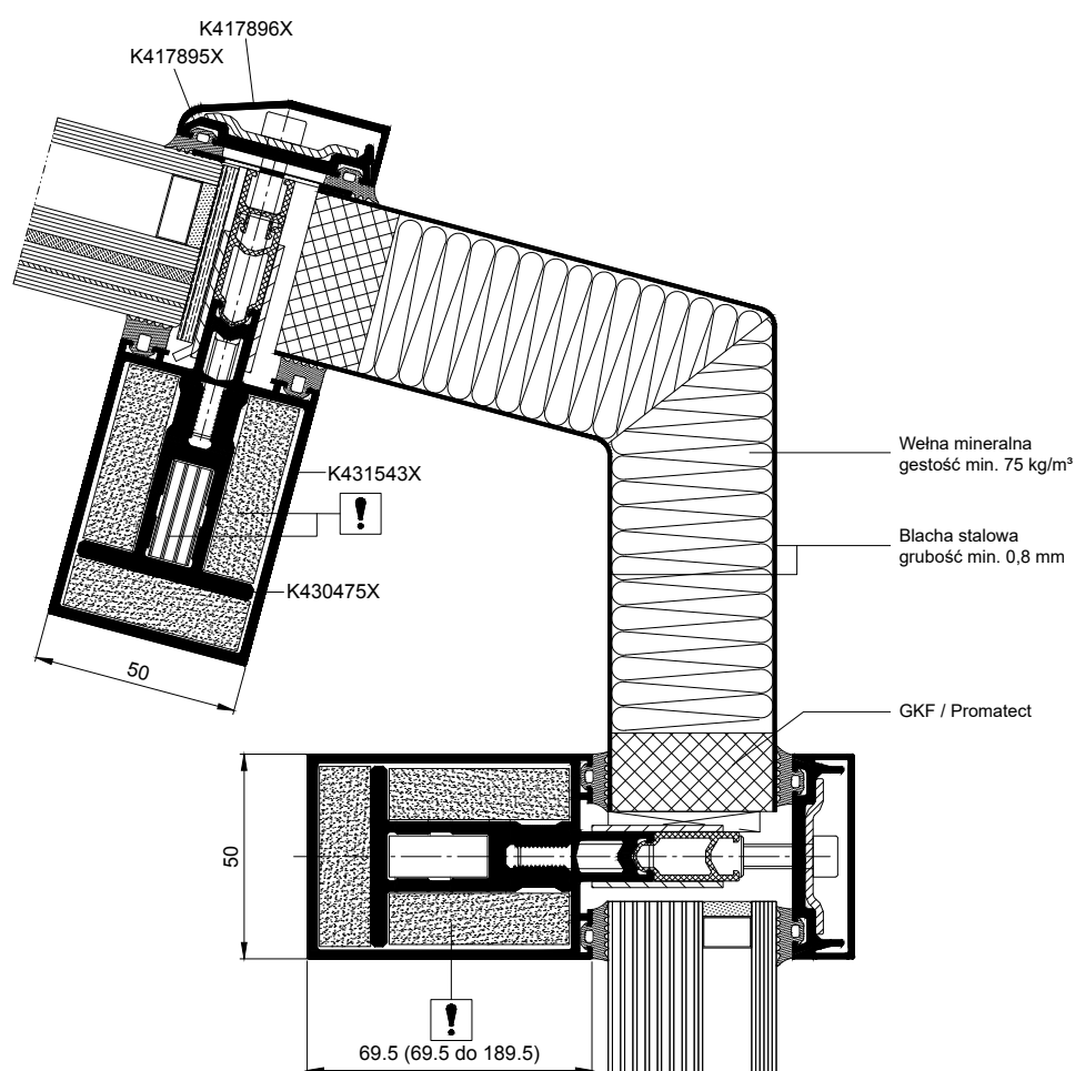
Przekrój przez połączenie dachu i fasady przeciwpożarowej
