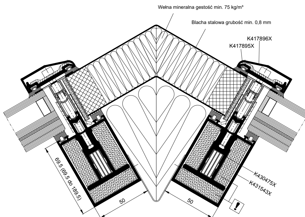
Przekrój przez połączenie dachu i fasady przeciwpożarowej
