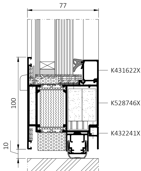
Przekrój dolny drzwi EI 60 bez progu
