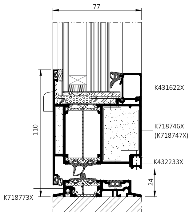
Przekrój dolny drzwi EI 30 z progiem
