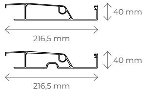
Przekrój pióra STANDARD (typ FLAT)
