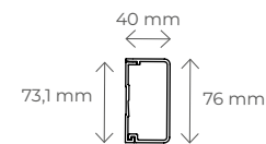
Przekrój prowadnicy
