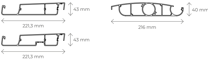
Przekrój belki z ukrytym silnikiem
