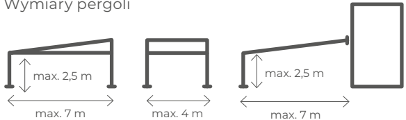
Wymiary pergoli
