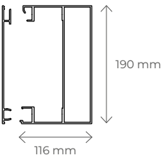
Przekrój belki
