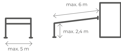
Wymiary pergoli
