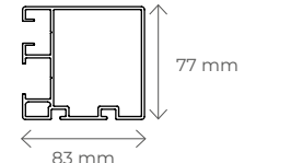
Przekrój prowadnicy
