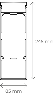
Przekrój belki z ukrytym silnikiem
