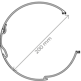
Przekrój słupa
