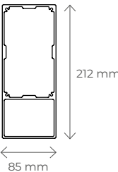
Przekrój belki z widocznym silnikiem
