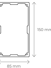
Przekrój słupa
