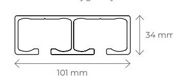
Przekrój prowadnicy dwutorowej górnej
